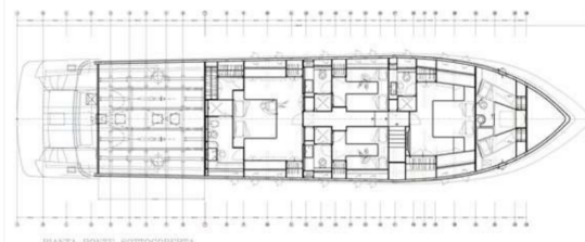
PIANTA PONTE SOTTOCOPERTA
